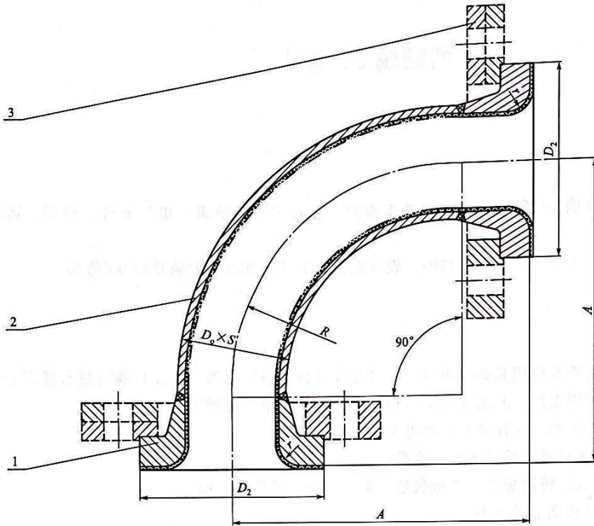
图 1 搪玻璃 90°弯头结构型式图
